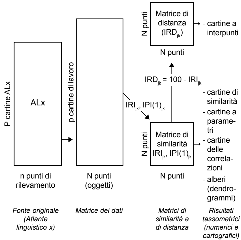
Figura 1: Schema della „catena dialettometrica“ AL: atlante linguistico IRI jk : Indice Relativo d’Identità IRD jk : Indice Relativo di Distanza IPI(1) jk : Indice Ponderato (col peso 1) d’Identità
